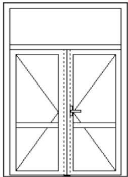
Pol.č.10 1610 x 2500; dveře O+O 1610 x 2100, nadsvětlík 1610 x 400
